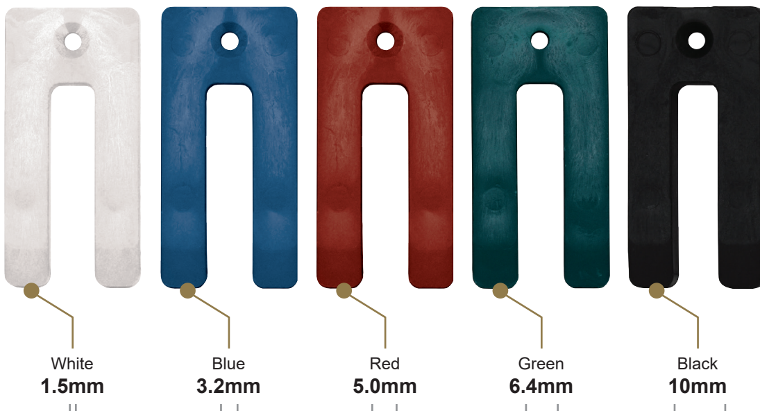
» Window spacing
